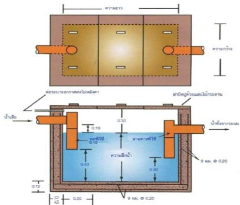
บ่อดักไขมันแบบสร้างในที่สำหรับอาคารขนาดใหญ่
