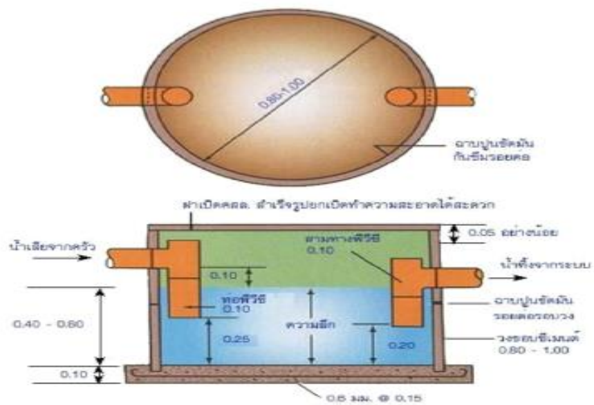
บ่อดักไขมันแบบวงขอบซีเมนต์สำหรับบ้านพักอาศัย
